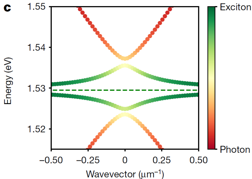
Polariton dispersion
