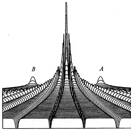
Potenziale quantico di Bohm
