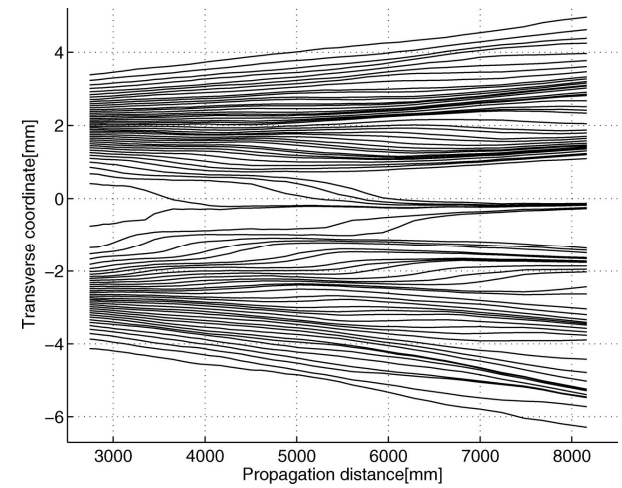
Misura "debole" su fotoni singoli
