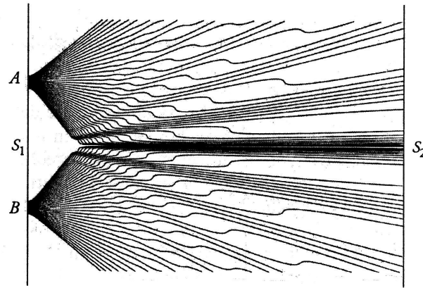
Traiettorie di Bohm
